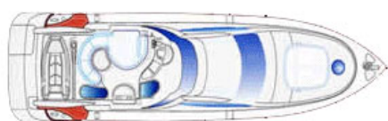
План флайбриджа
